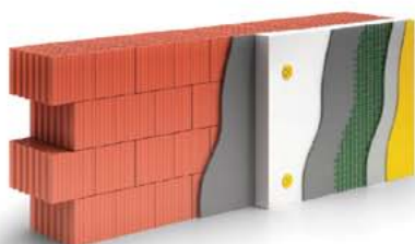
Стена из керамических блоков 380 мм с утеплителем ППС и штукатурная отделка
